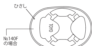
※TOYOの刻印を前側 (図-3)
